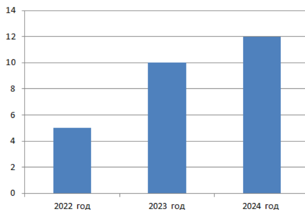
Рис. 3. Диаграмма уборки береговой линии Байкала
